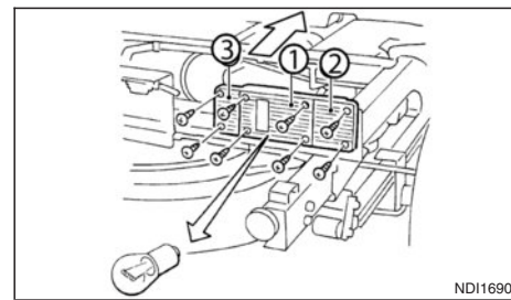
Bloc optique arrière (clignotant, stop et feu de recul) (modèles sans benne) NDI1690
