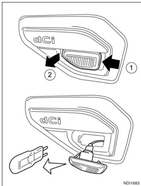
Clignotant latéral (aile sur l'aile avant) (selon modèles) NDI1683
