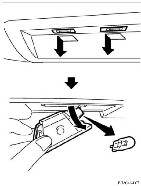
Kennzeichenleuchte
